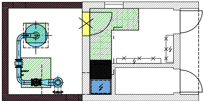
Grundriss Erdgeschoss
